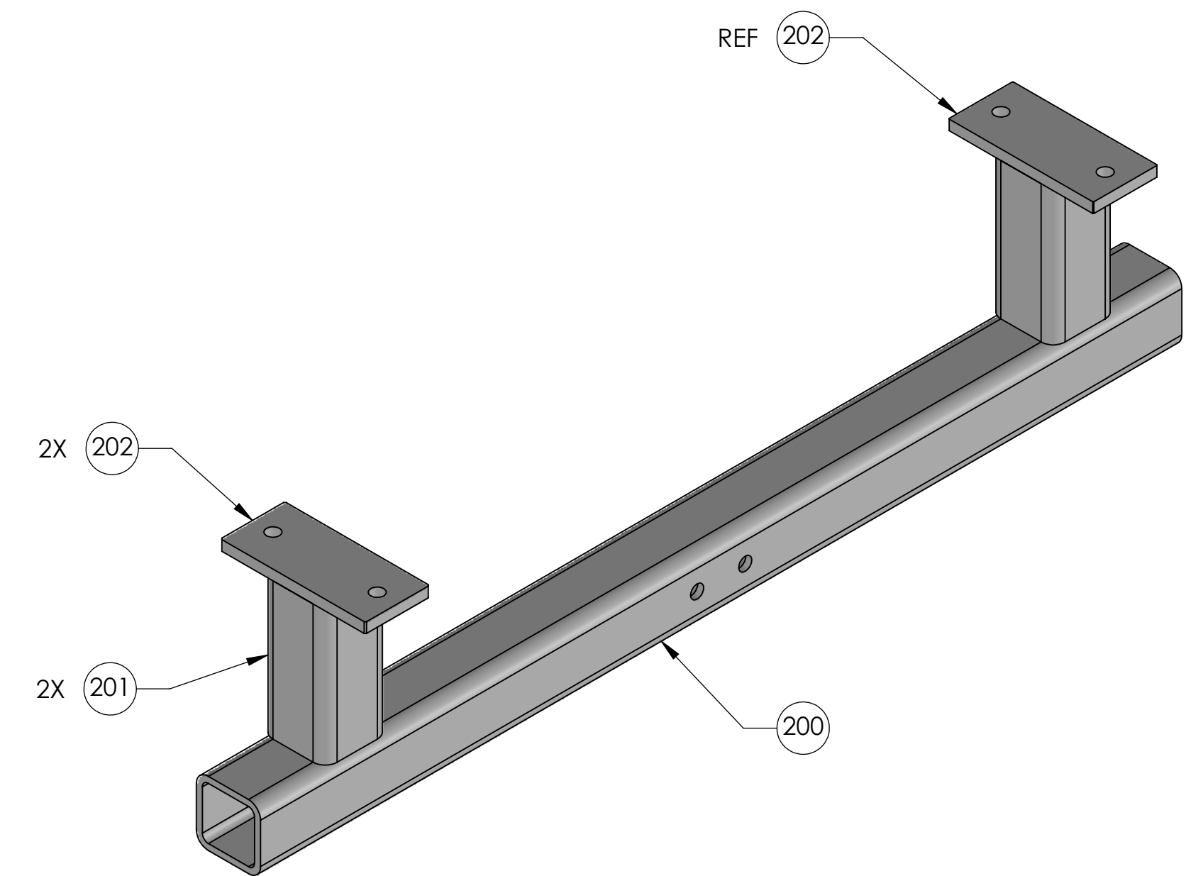
ITEM 2 SCALE 1 : 6
