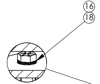
DETAIL B SCALE 1 : 1 3 PL.
