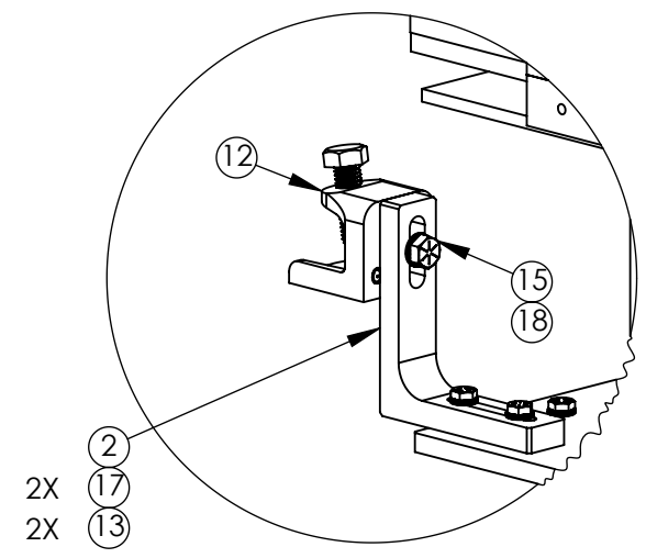
DETAIL A SCALE 1 : 4 2 PL.
