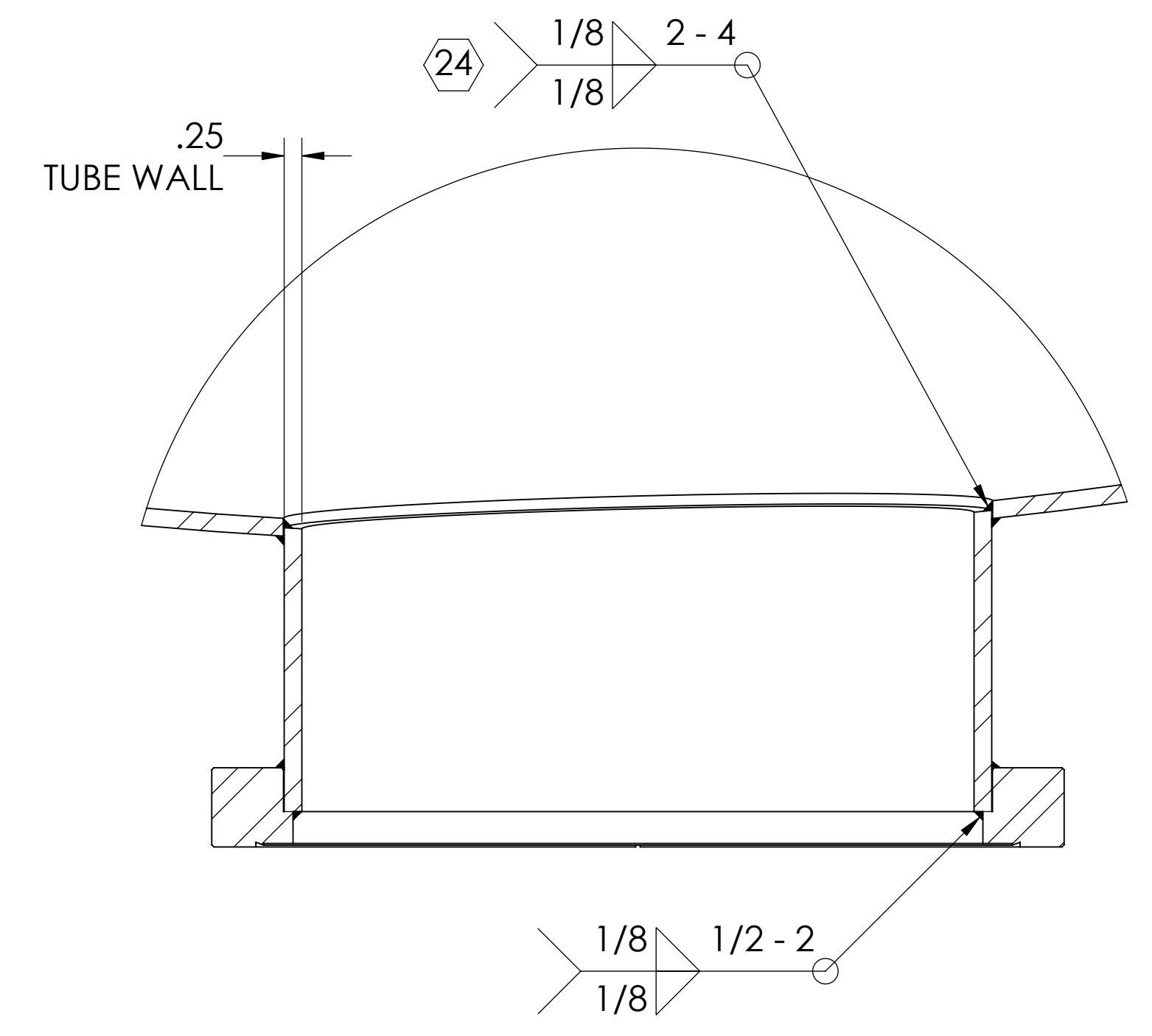
DETAIL K SCALE 1 : 2 2 PL.
