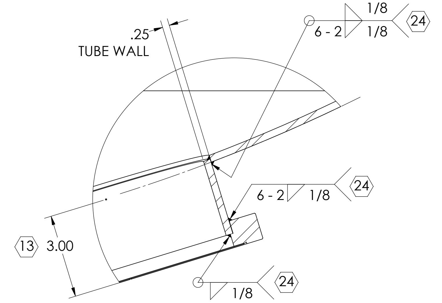
DETAIL D SCALE 1 : 2 3 PL.
