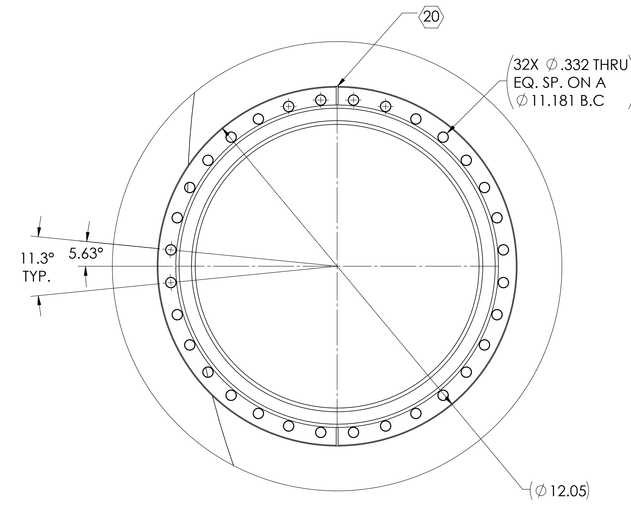
DETAIL E SCALE 1 : 2 2 PL.
