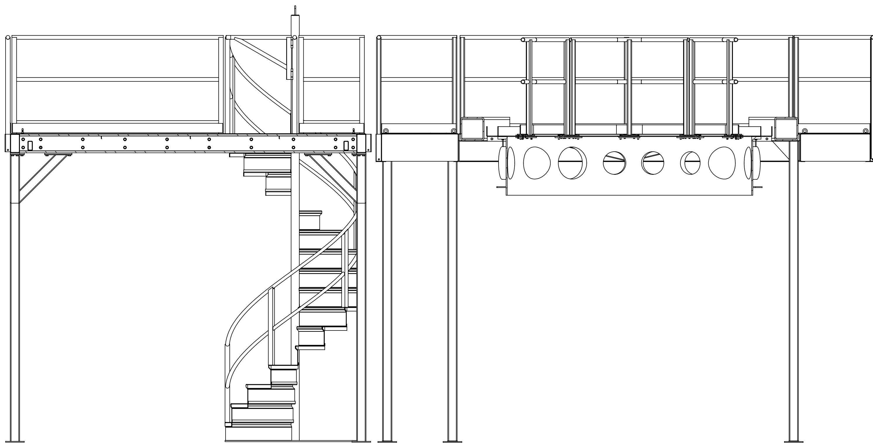
SECTION B-B SCALE 1 : 24
