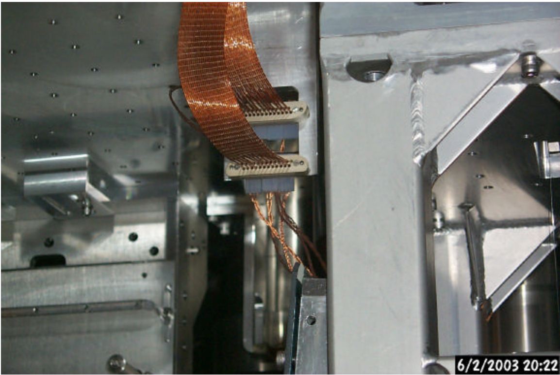
New 2k ITMx OSEM connector.
