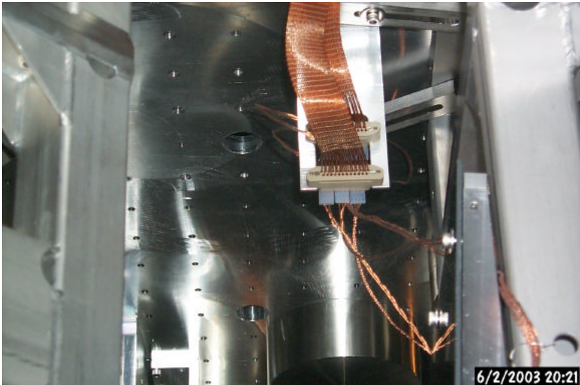
New 2k ITMx LOS OSEM connector.
