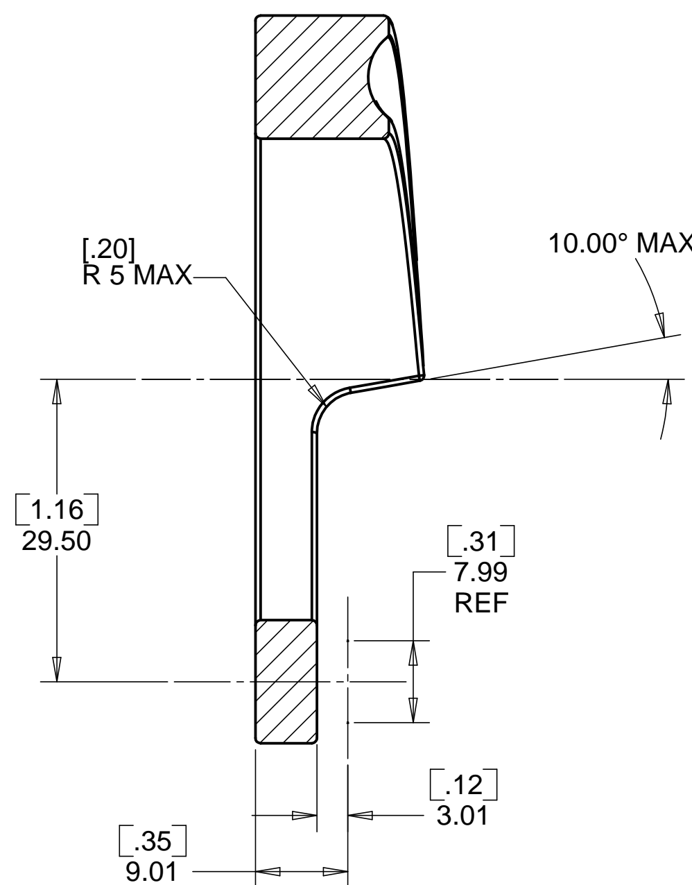
SECTION A-A SCALE 2 : 1
