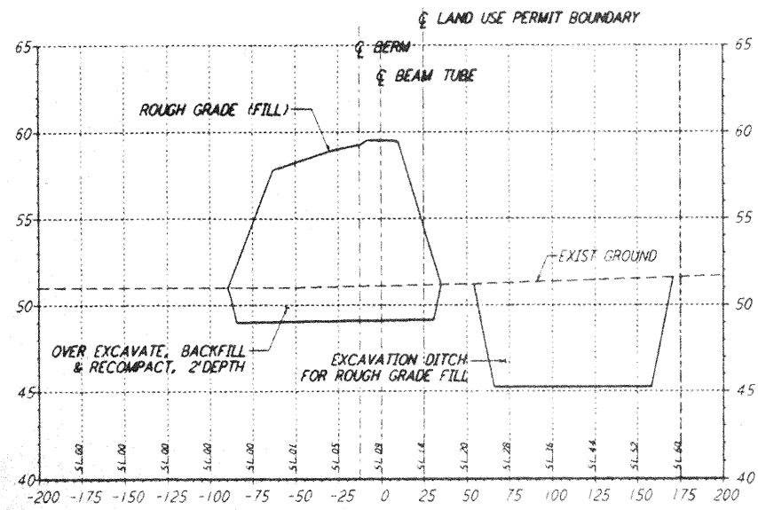
STA 130+00.00
