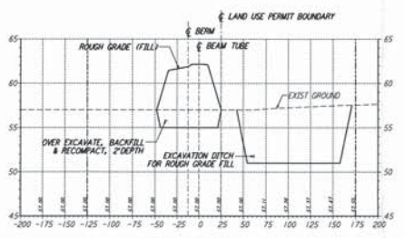
STA 26+00.00
