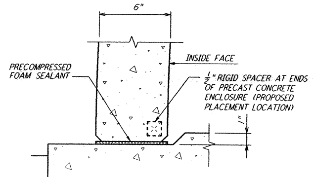
DETAIL 7 3'' = 1'-0''
