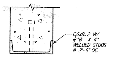
DETAIL 8 3'' = 1'-0''
