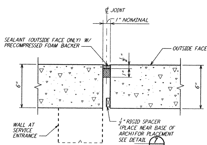
DETAIL 6 3'' = 1'-0''
