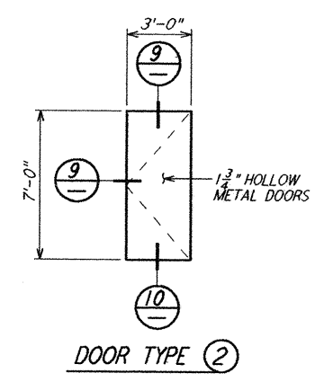
DOOR TYPES NTS
