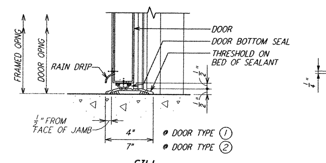
SILL DETAIL 10 3'' = 1'-0''
