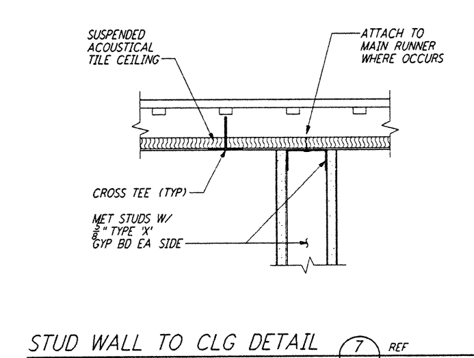
STUD WALL TO CLG DETAIL
