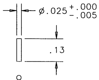
-2. GUIDE ROD SCALE: 4/1
