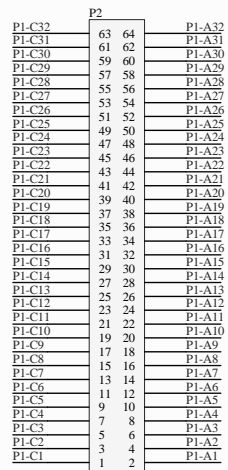
HEADER 32X2
