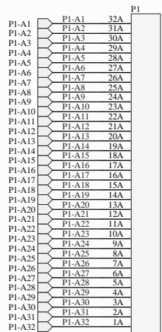
DIN96
