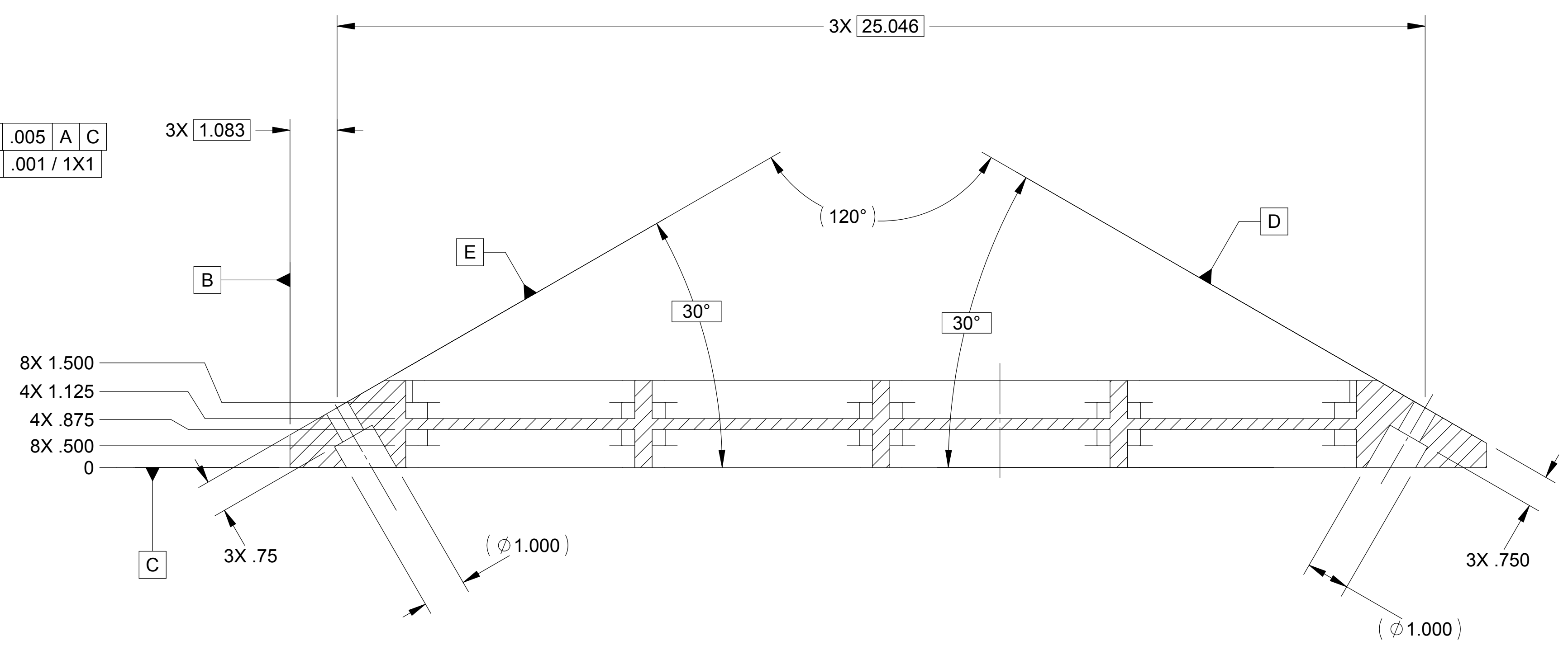
SECTION D-D
