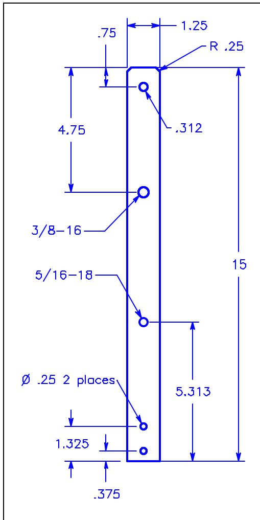
Strap
